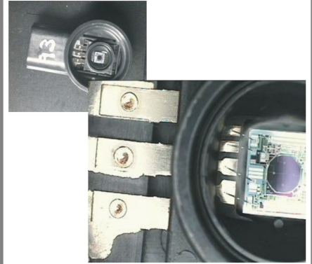
引擎温度传感器的焊接
